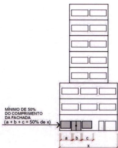
ELEVÇÃO FACHADA ATIVA - MEIO DE QUADRA S/ ESCALA
