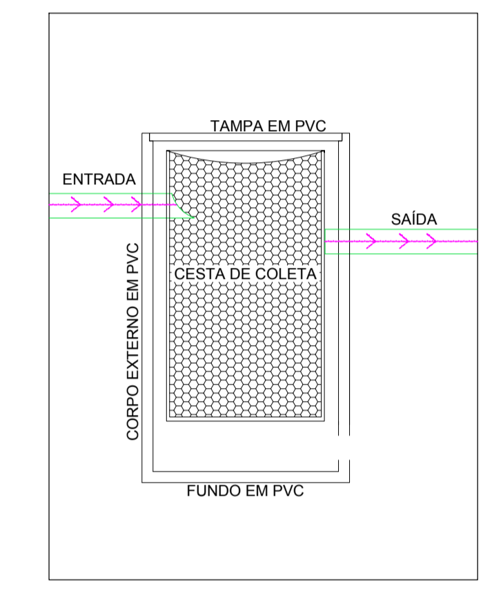
DETALHE CAIXA DE GORDURA 20L fora de escala
