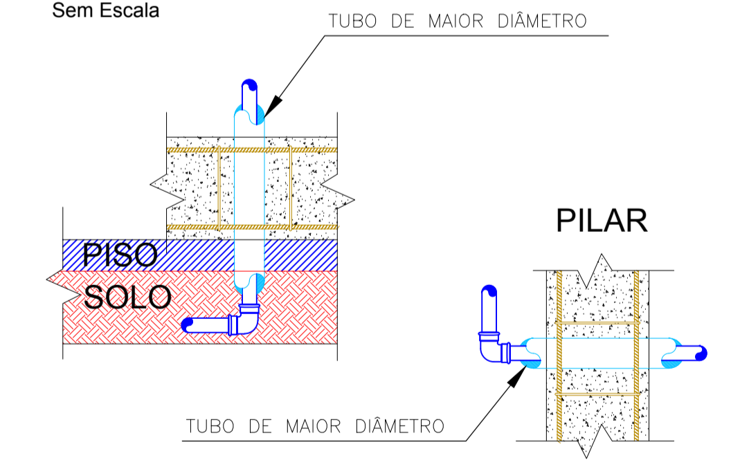
DETALHE 01 PASSAGEM POR VIGAS/PILARES E PISOS Sem Escala
