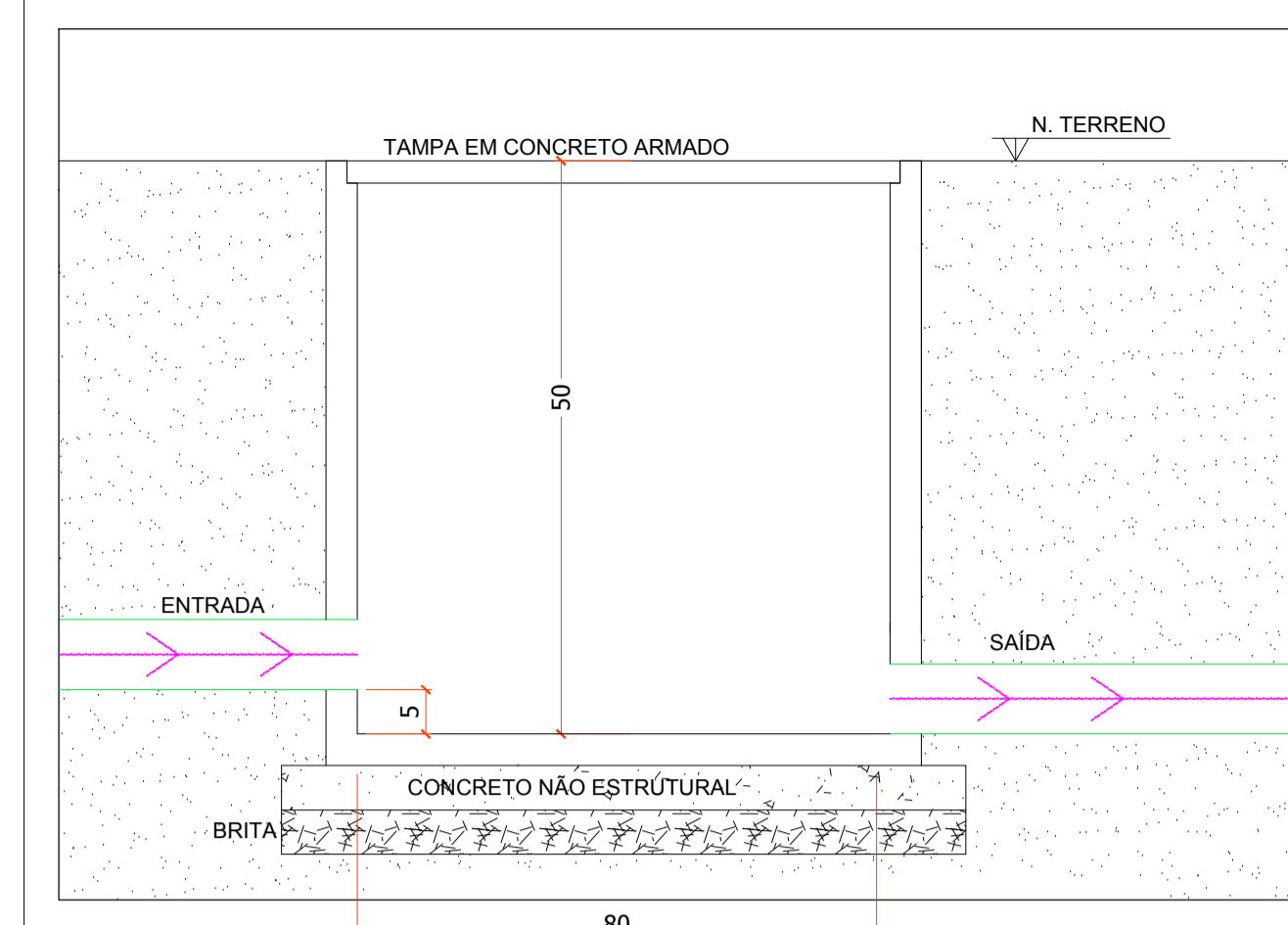
DETALHE CAIXA DE INSPEÇÃO fora de escala
