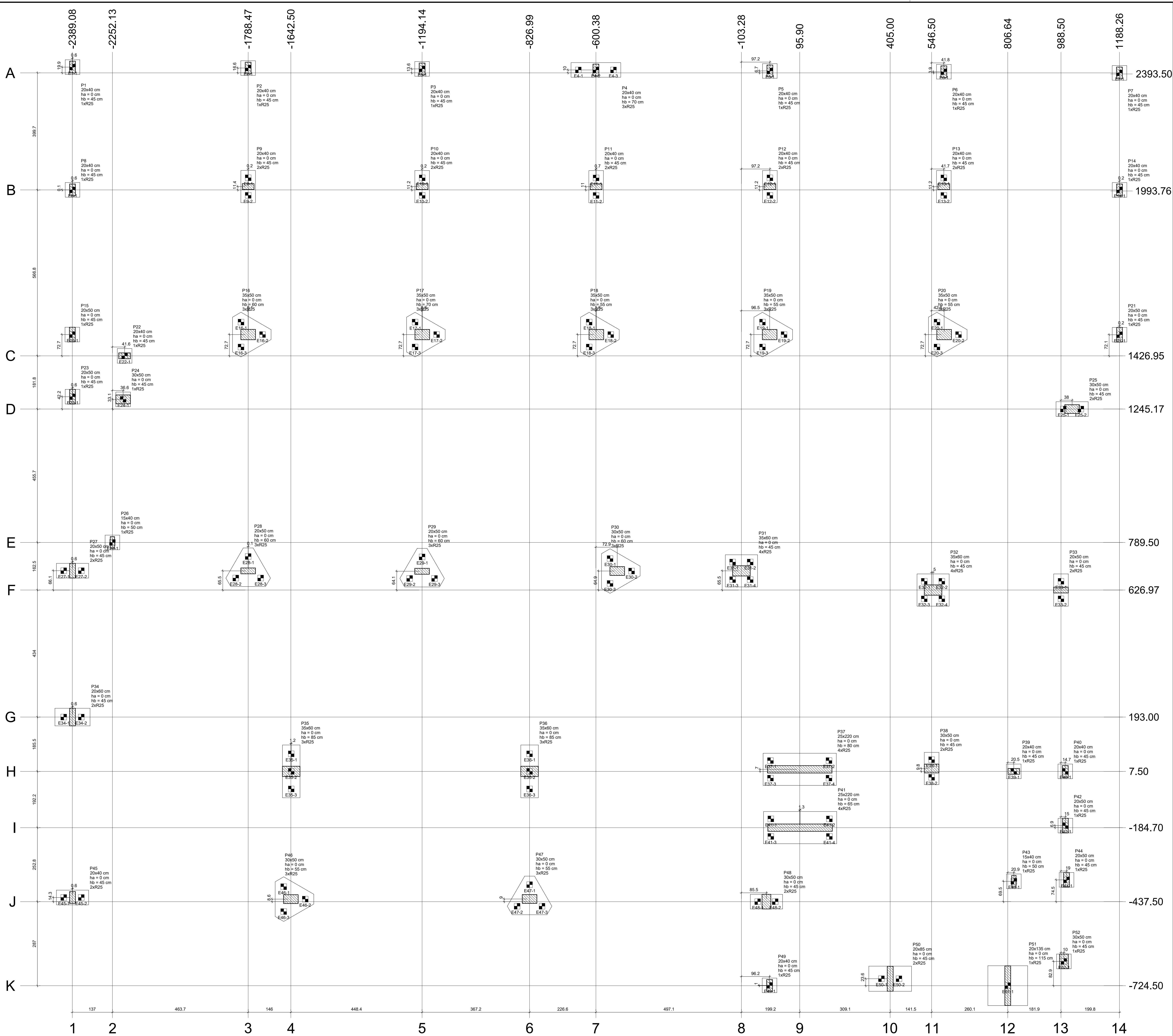
LOCAÇÃO DE ESTACAS Escala 1:50
