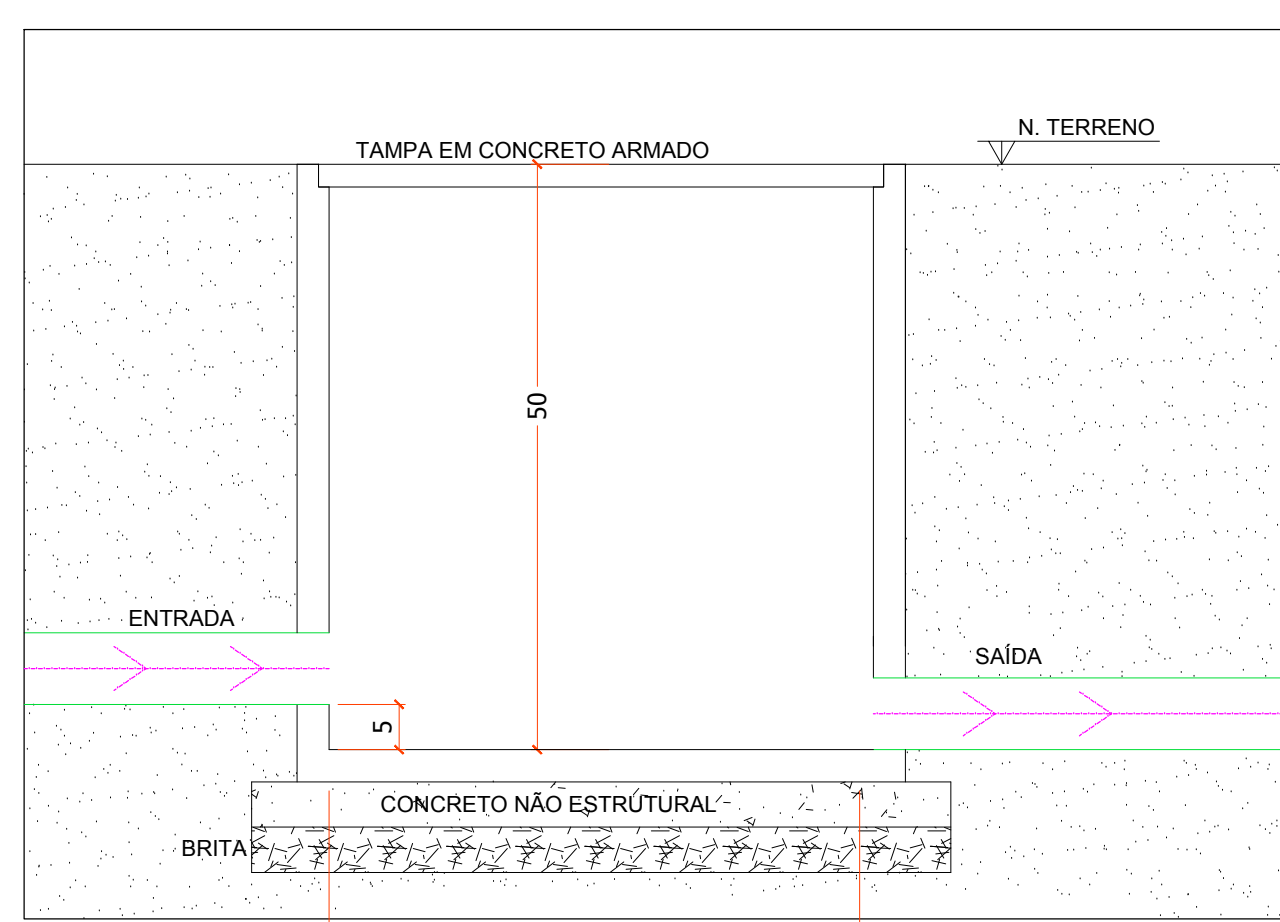
DETALHE CAIXA DE INSPEÇÃO fora de escala
