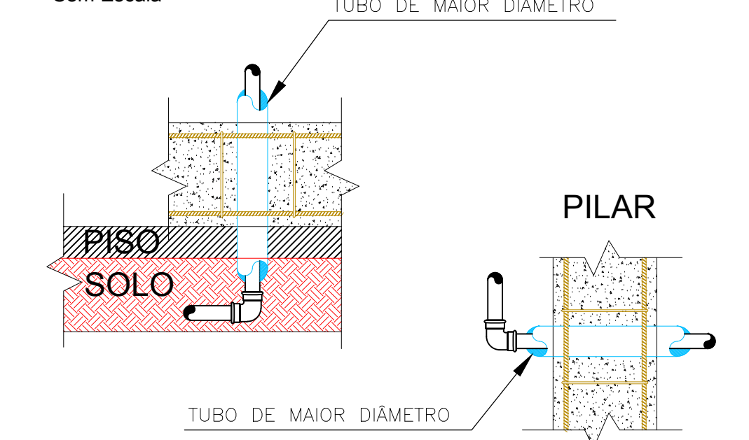
DETALHE 01 PASSAGEM POR VIGAS/PILARES E PISOS Sem Escala
